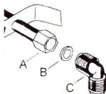
A) Fim do trem de gás com porca B) Gaxeta C) União ajustável
